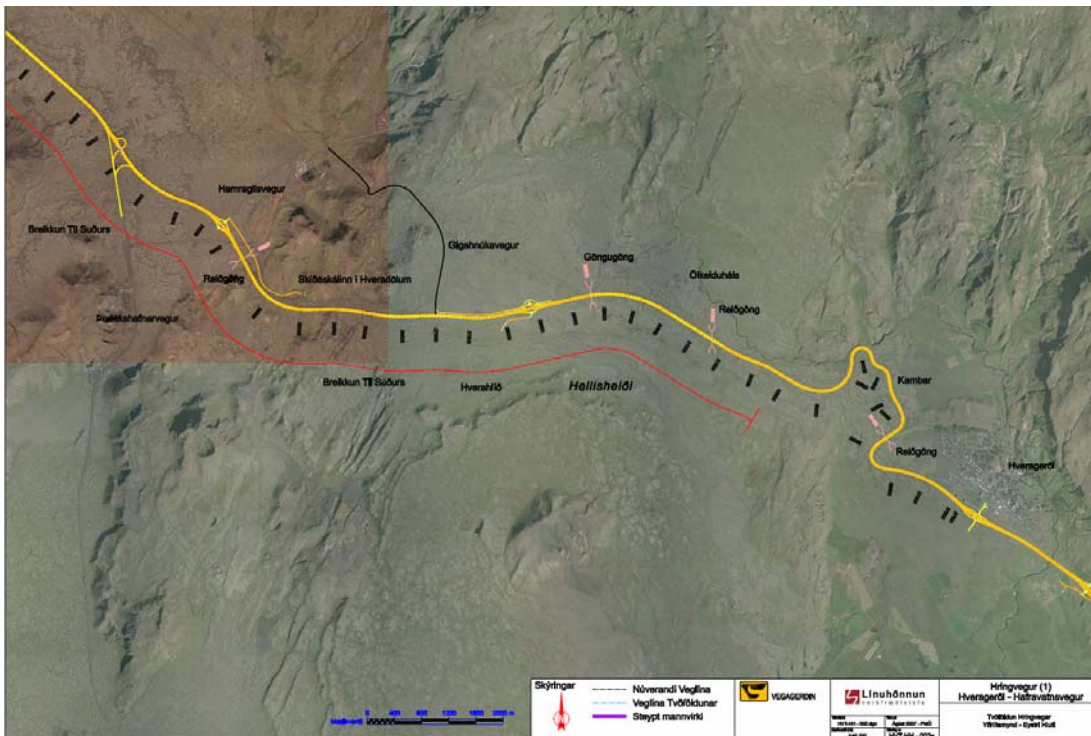
Mynd 2-2 Yfirlitsmynd tvöföldun Suðurlandsvegur – Hellisheiði að Hveragerði.
